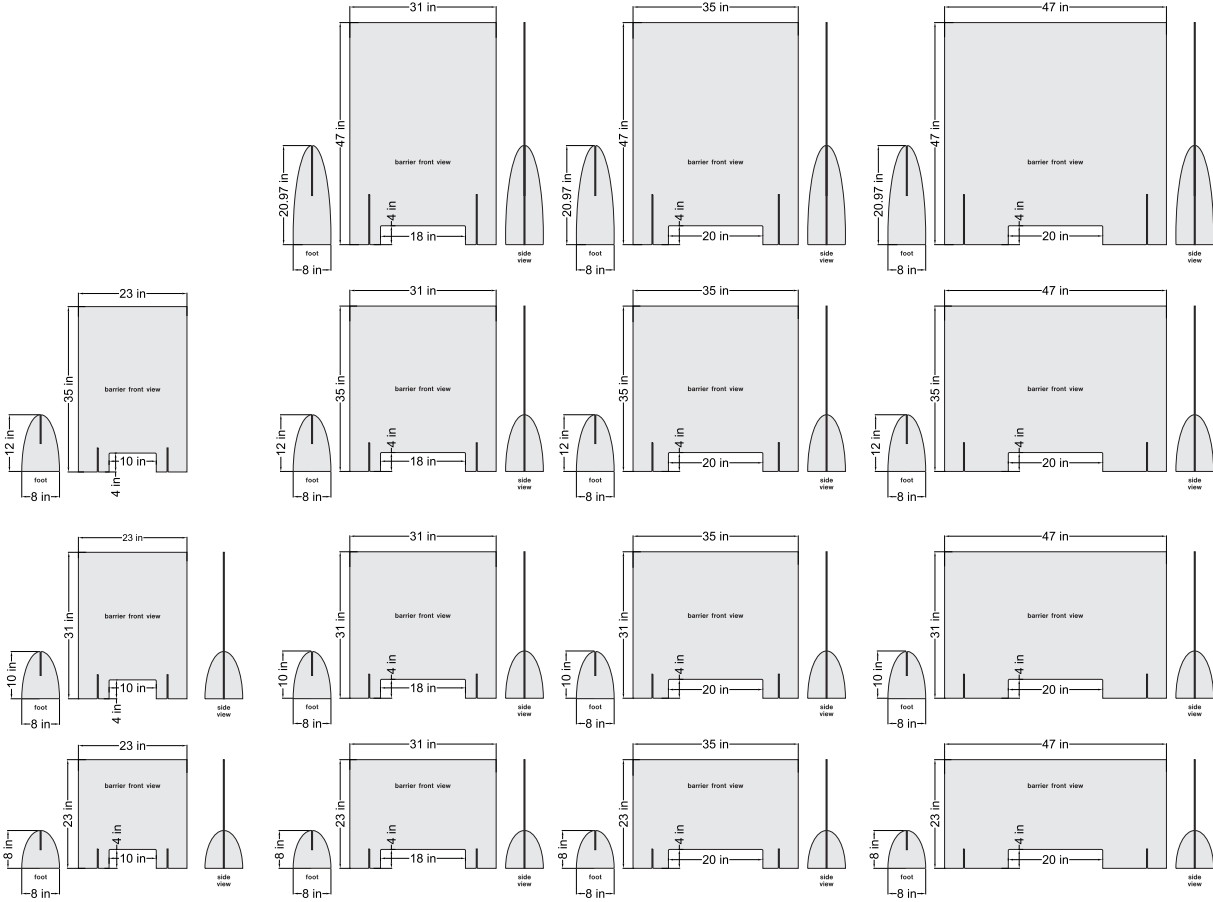
Optional bent foot
